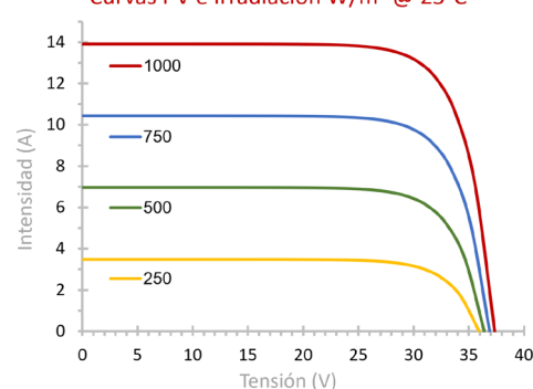
Curvas I-V e Irradiación W/m 2 @ 25°C
