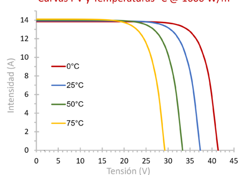
Curvas I-V y Temperaturas °C @ 1000 W/m 2
